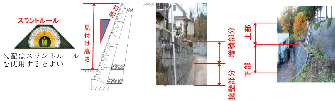
(a)一般の擁壁高さ（見付け高さ） (b)増積み擁壁の高さ (c)二段擁壁の高さ
